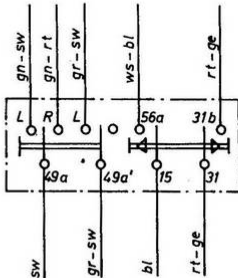
BLH (Lenksäulenschalter)
