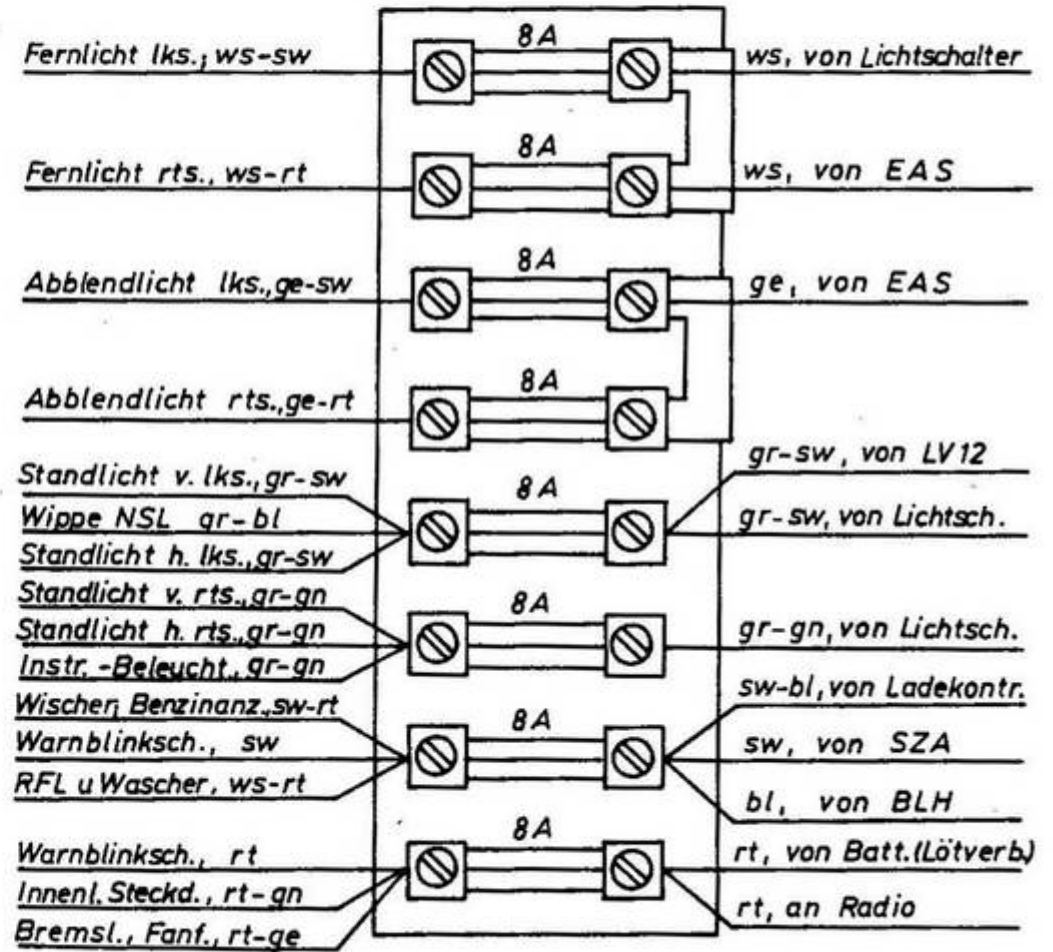
Si 1...8 (Sicherungsdose)
